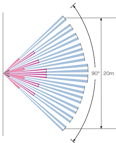
Padrão da lente - vista de cima
